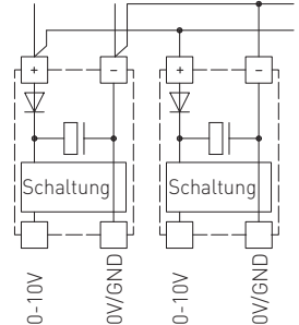
4-Leiter- Anschluss PREMASGARD® 722x
