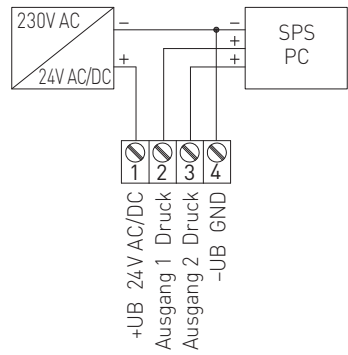
4-Leiter- Anschluss PREMASGARD® 722x
