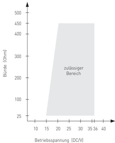
Bürendiagramm (4...20 mA) PREMASGARD® 722x
